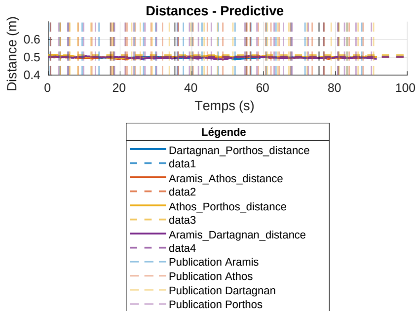
FIGURE 7.17 – Evolution des inter-distances entre les robots
