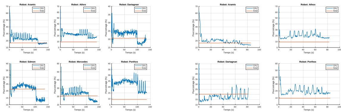
(7.20.1) Méthode classique
