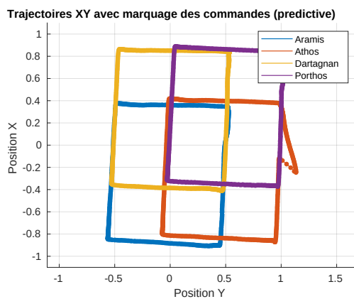
FIGURE 7.18 – Trajectoire des robots avec une perturbation
