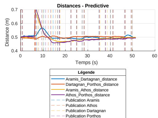
FIGURE 7.19 – Evolution des inter-distances entre les robots avec perturbation
