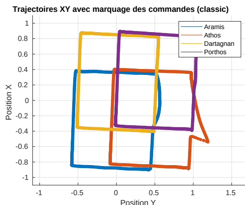
FIGURE 7.5 – Trajectoire des robots avec une perturbation
