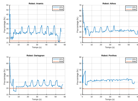
(7.22.1) Pourcentage CPU et RAM utilisé (Classique)
