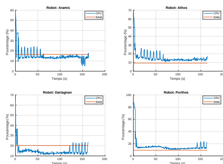
(7.22.5) Pourcentage CPU et RAM utilisé (Prédictive)
