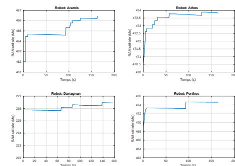
(7.22.6) Quantité de RAM utilisée (Prédictive)
