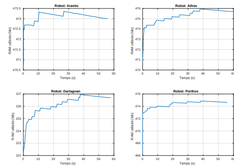
(7.22.2) Quantité de RAM utilisée (Classique)
