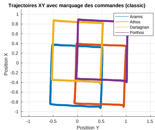
FIGURE 7.3 – Trajectoire de chaque robot de l'essaim
