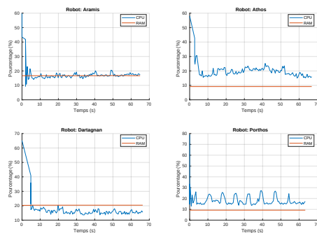
(7.22.3) Pourcentage CPU et RAM utilisé (Événementielle)
