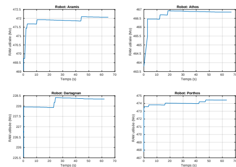
(7.22.4) Quantité de RAM utilisée (Événementielle)
