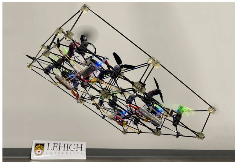
FIGURE 2.1 – Système ModQuad [4].
