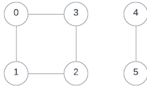
FIGURE A.4 – Exemple 2 de graphe non connexe
