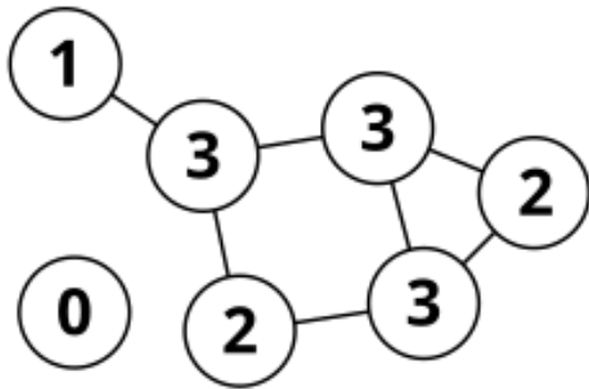
FIGURE A.3 – Exemple 1 de graphe non connexe
