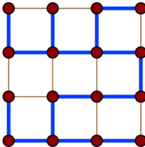
FIGURE A.5 – Exemple d'un arbre couvrant (en bleu)
