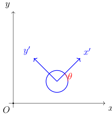
FIGURE 6.3 – Repères 2D : global (x, y) et repère body (x', y') tourné de l'angle \theta . Le cercle représente le robot.
