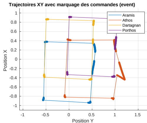
FIGURE 7.13 – Trajectoire des robots avec une perturbation
