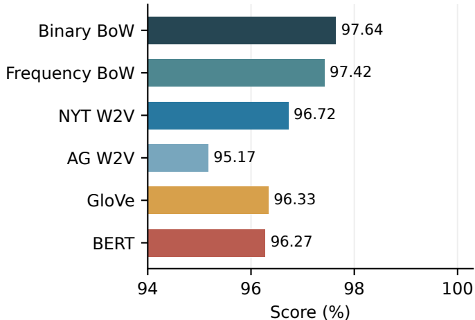
(b) Macro-F1
