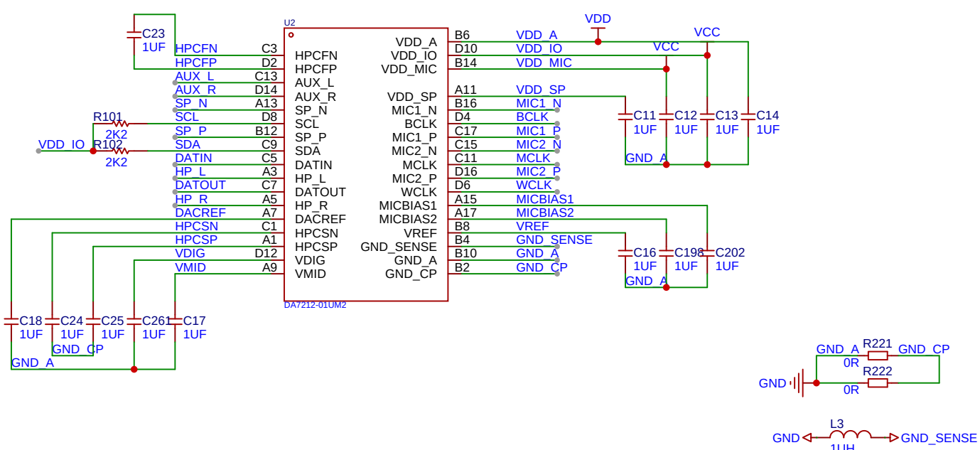
DA7212
