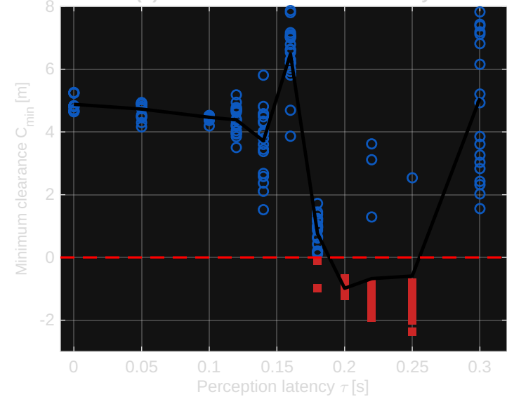
(d) Minimum clearance vs. latency
