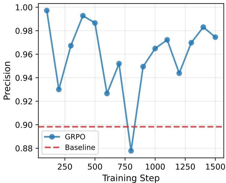
(d) Precision
