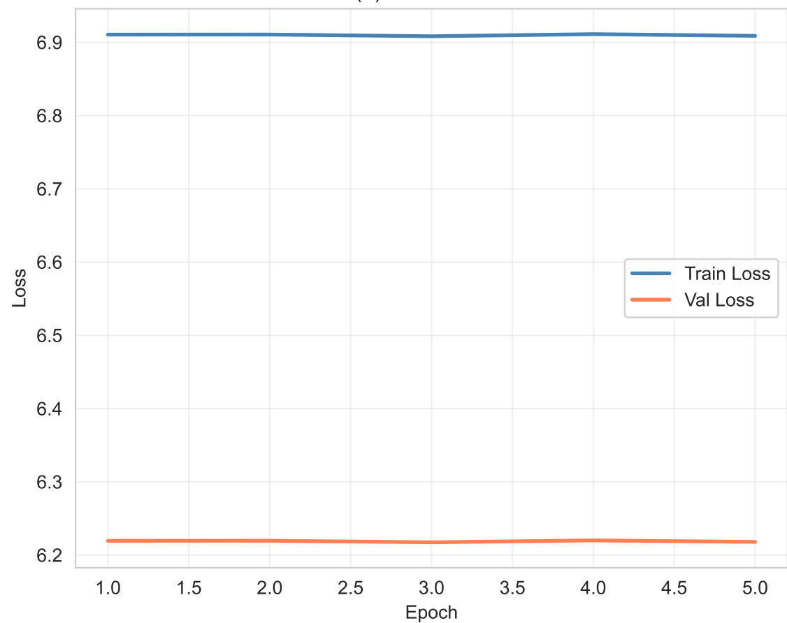
(d) CTC
