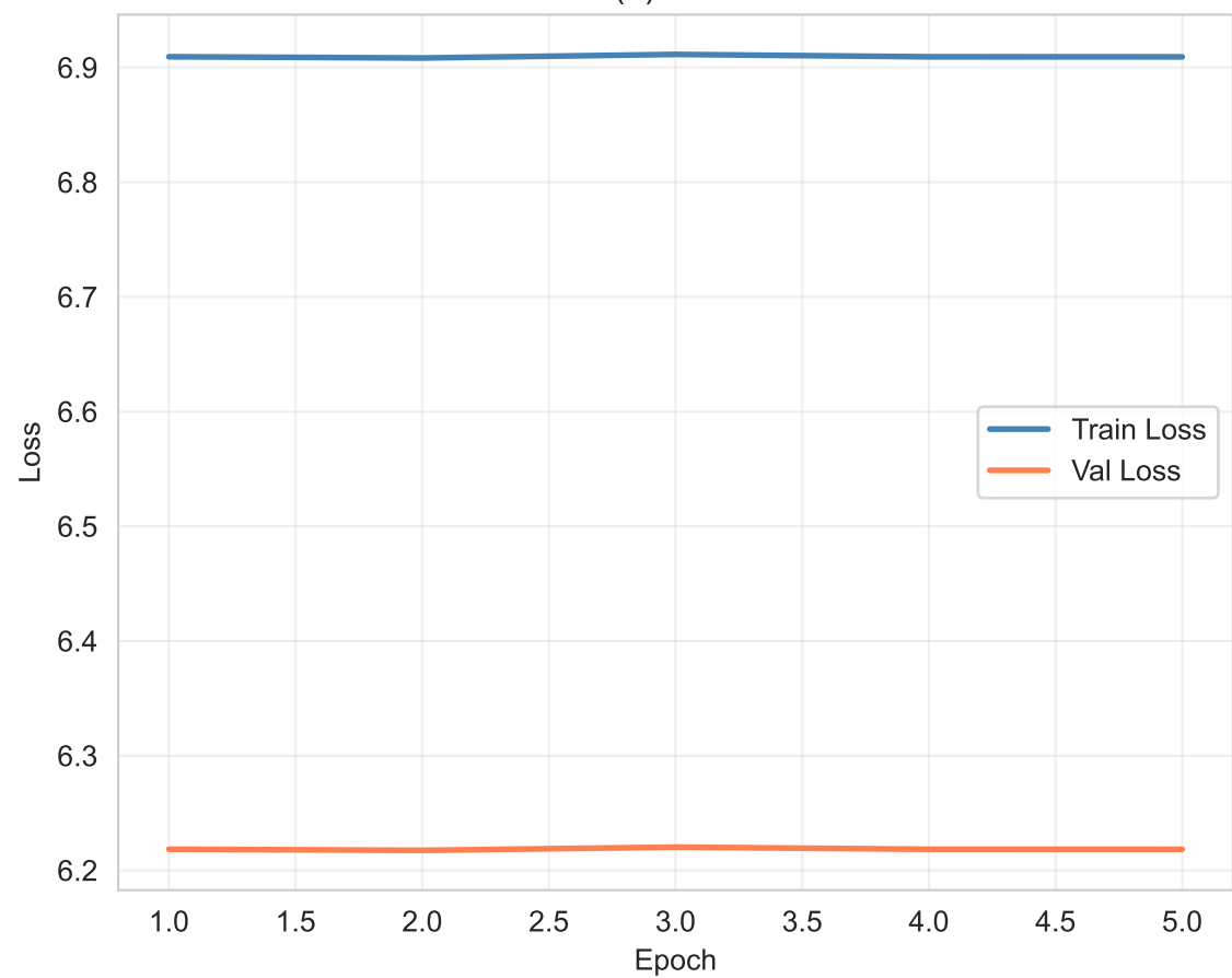
(d) CTC
