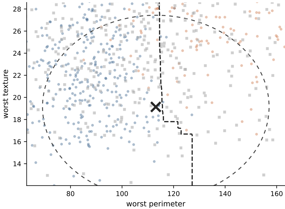
C · perturbation
