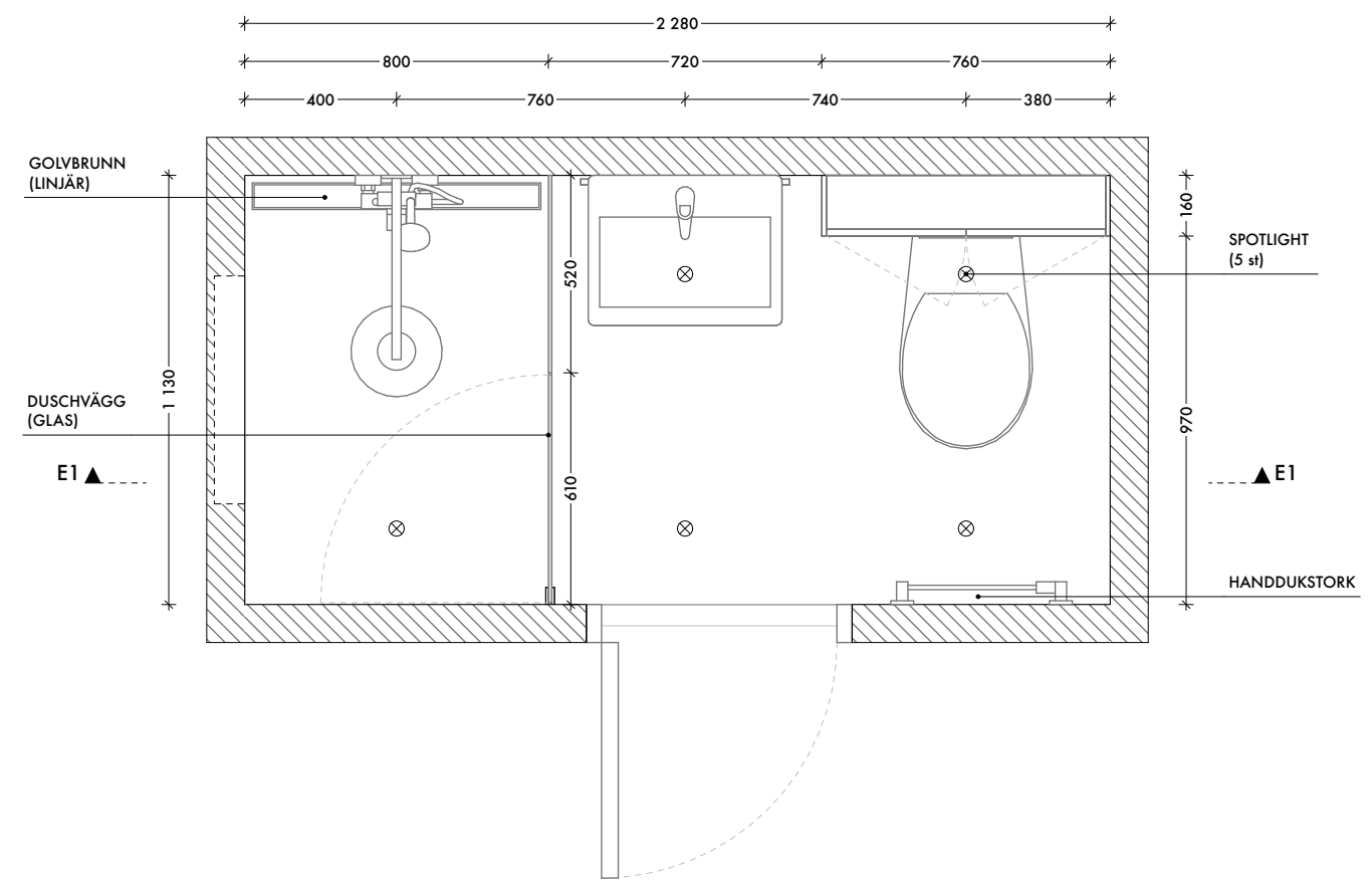
PLAN 1:20
