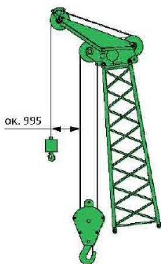
Главная стрела SHLH с гуськом S12.1 (12 т)
