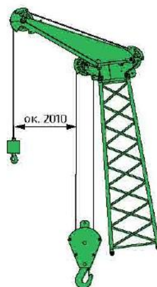
Главная стрела SHLH с гуськом S24.1 (24 т)
