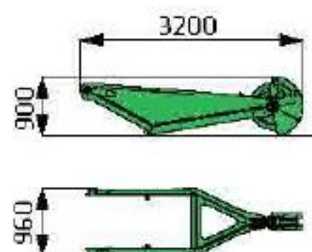
Гусек S12.1 (370 кг) грузоподъемность 12,0 т
