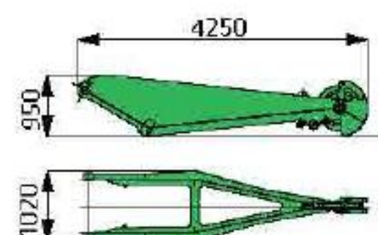
Гусек S24.1 (510 кг) грузоподъемность 24,0 т
