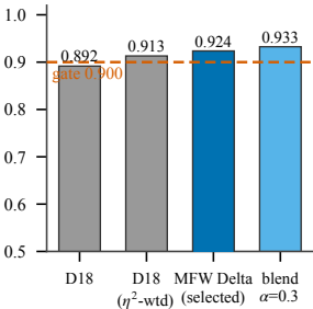
E1 separation AUC
