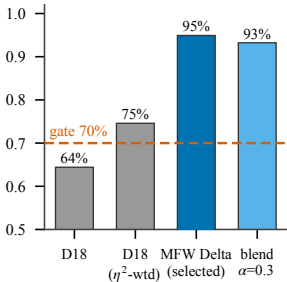
E2 top-1 attribution
