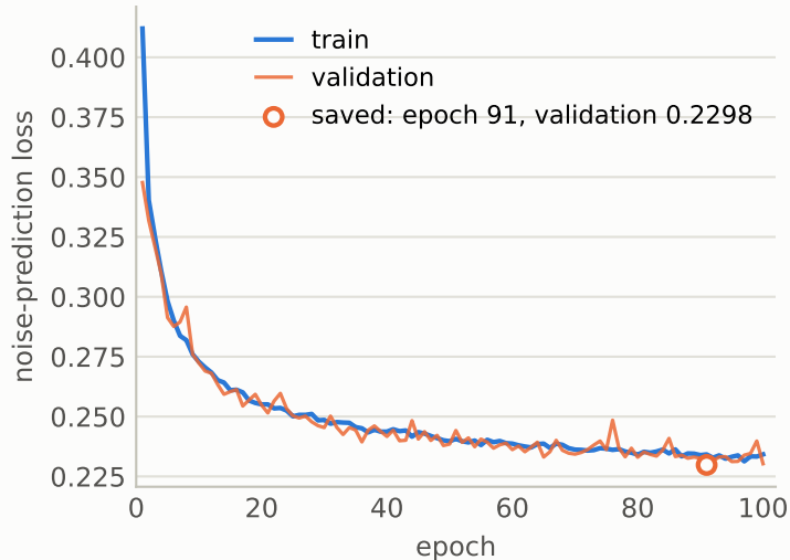
Diffusion
