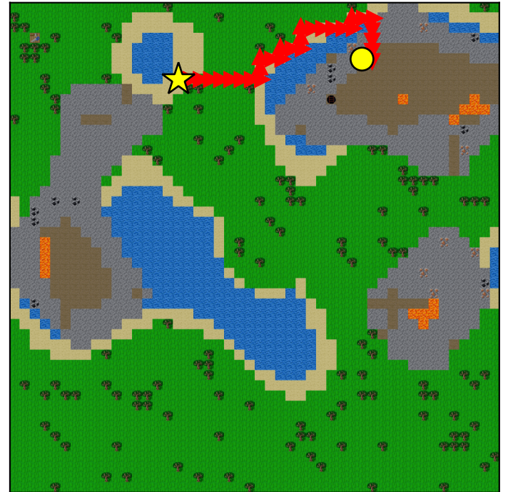
Test
