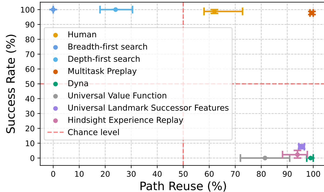
Threshold = 0.7
