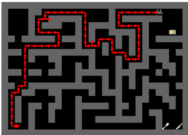
Eval | start_pos=[17 1]
