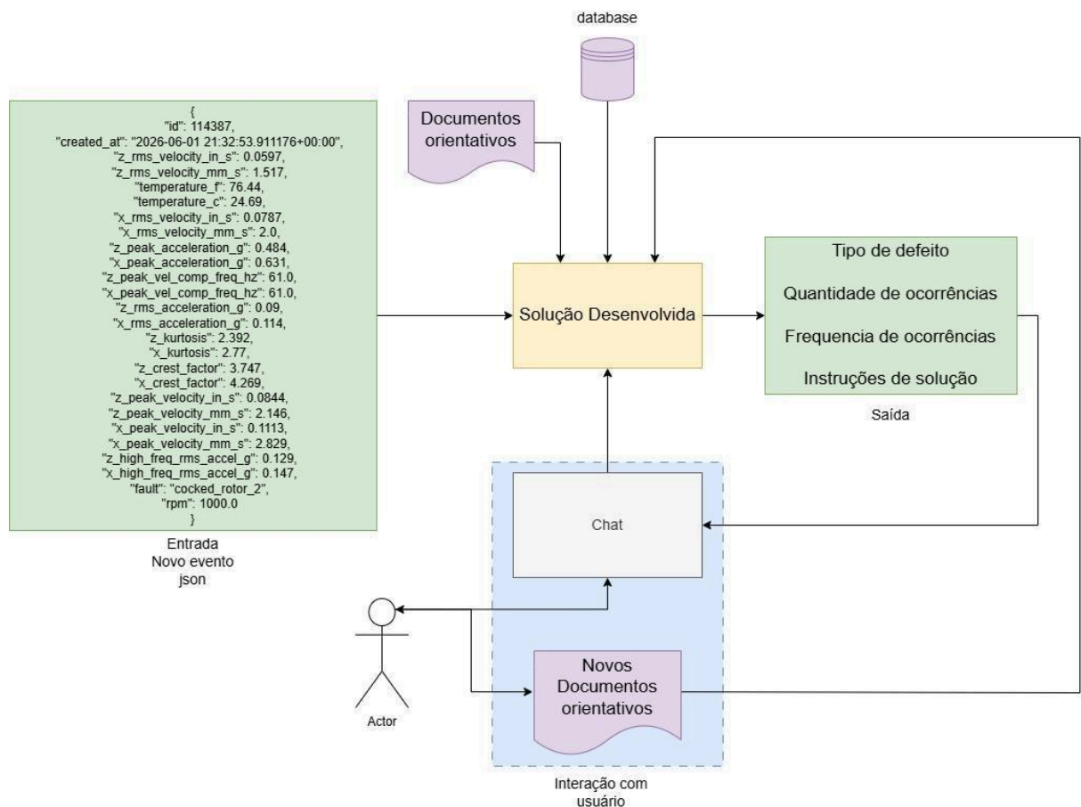
Figura 01 - Diagrama Geral das funcionalidades esperadas para a solução
