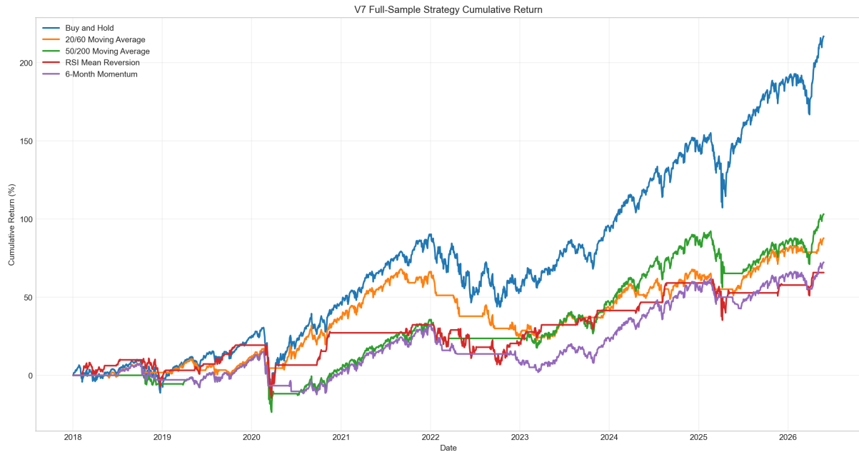
v7_strategy_comparison_full.png
