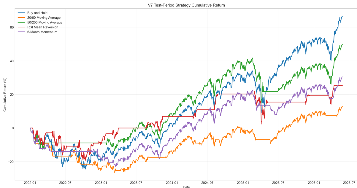
v7_strategy_comparison_test.png
