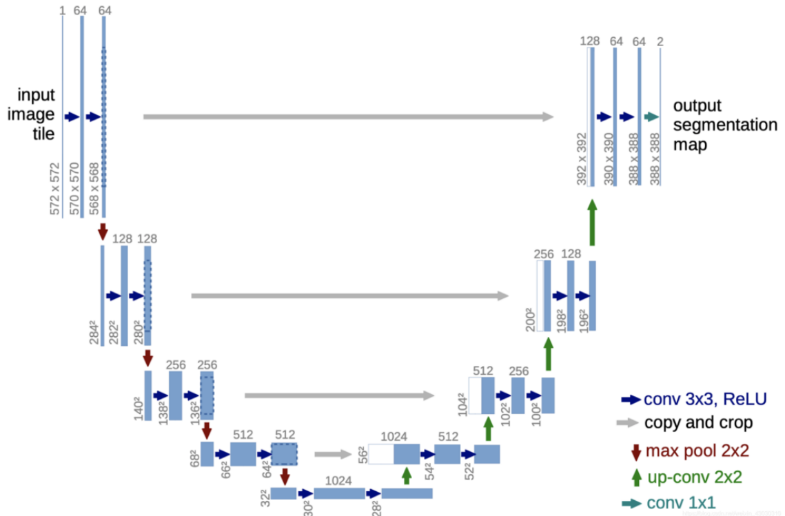
图 4.1 U-Net 网络架构图 [10]
