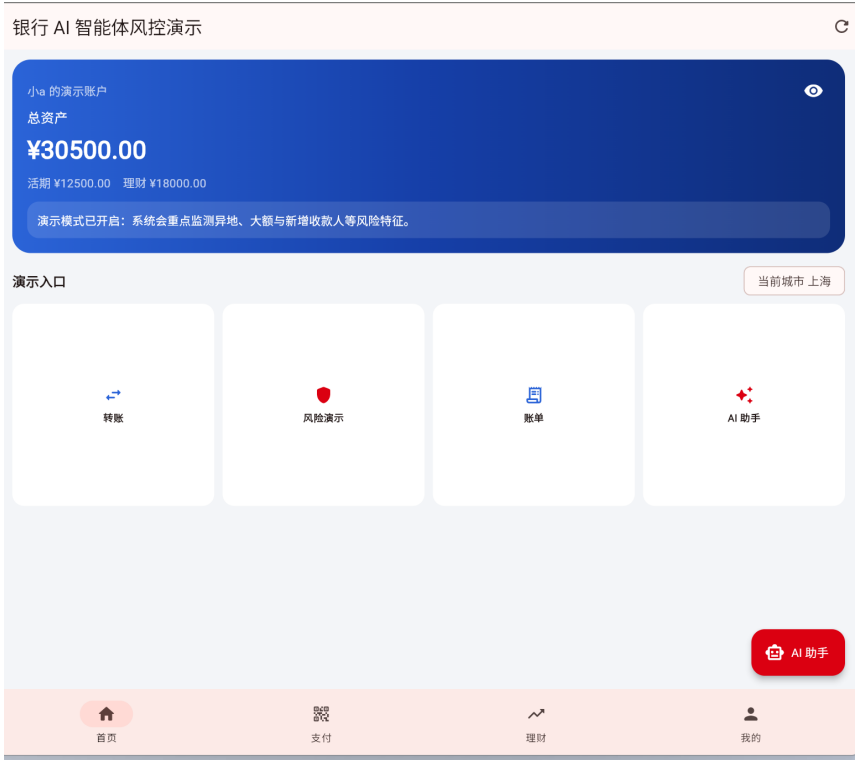
图 4.1 首页
