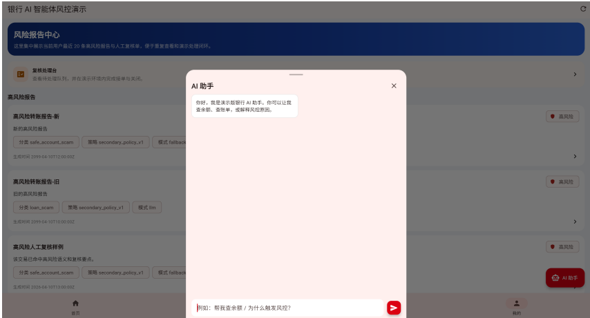
图 4.5 AI 助手
