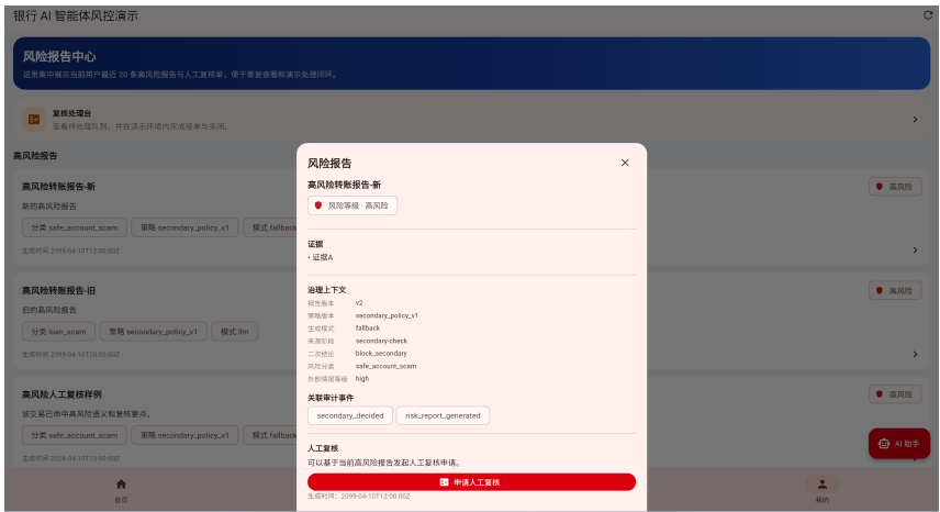
图 4.4 风险报告
