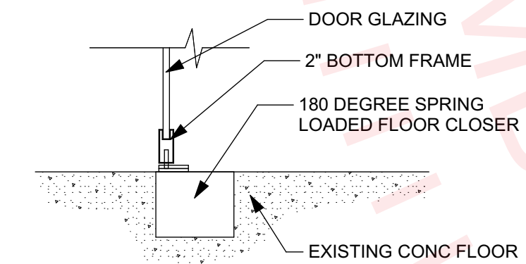
7 A-603 DOOR SILL SCALE: 1 1/2" = 1'-0"
