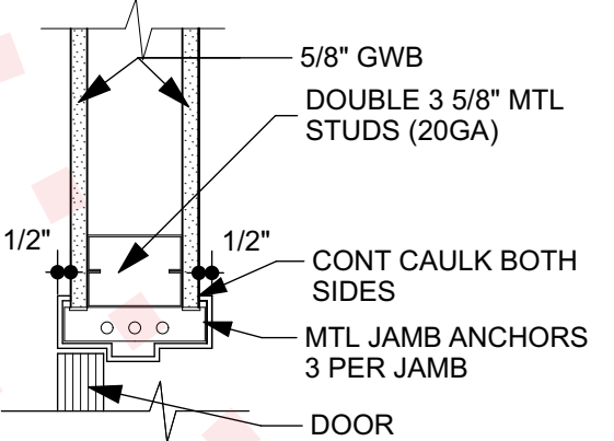
5 A-601 DOOR JAMB SCALE: 1 1/2" = 1'-0"
