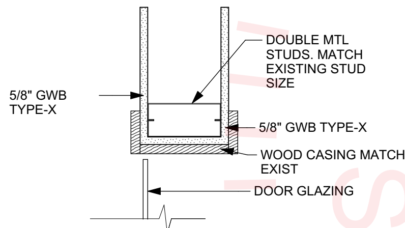
8 A-603 DOOR JAMB SCALE: 1 1/2" = 1'-0"
