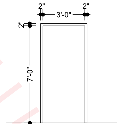
3 A-601 Door Frames SCALE: 1/4" = 1'-0"
