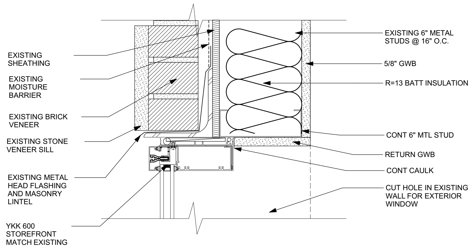
7 A-602 EXTERIOR WINDOW HEAD SCALE: 3" = 1'-0"
