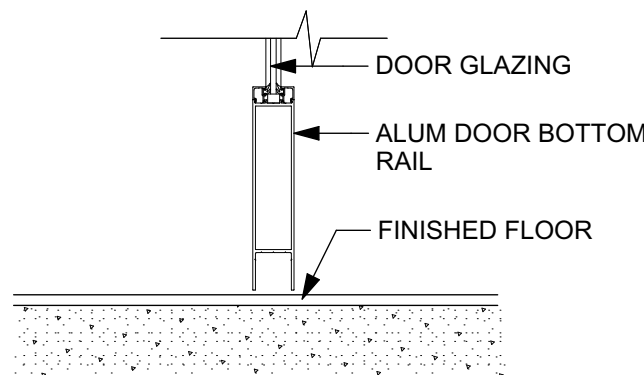
10 A-601 DOOR SILL SCALE: 1 1/2" = 1'-0"
