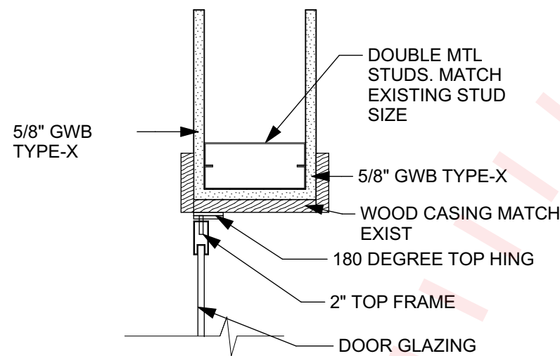
9 A-603 DOOR HEAD SCALE: 1 1/2" = 1'-0"
