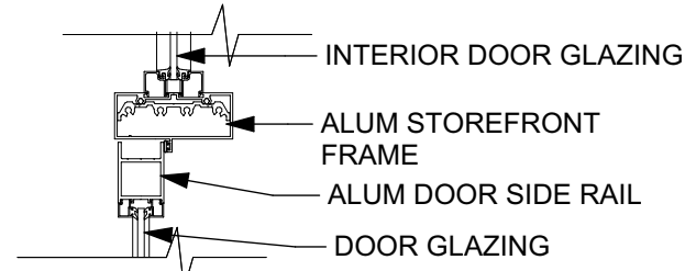
11 A-601 DOOR JAMB SCALE: 1 1/2" = 1'-0"
