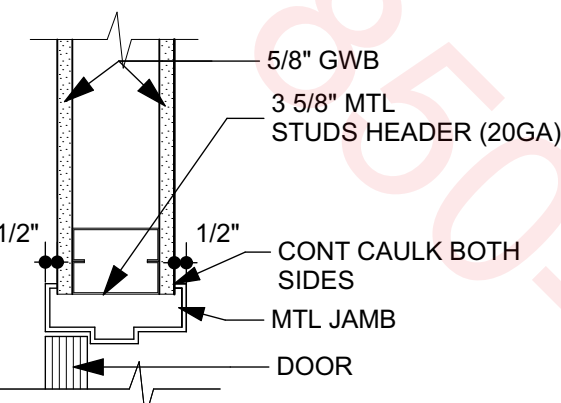
6 A-601 DOOR HEAD SCALE: 1 1/2" = 1'-0"
