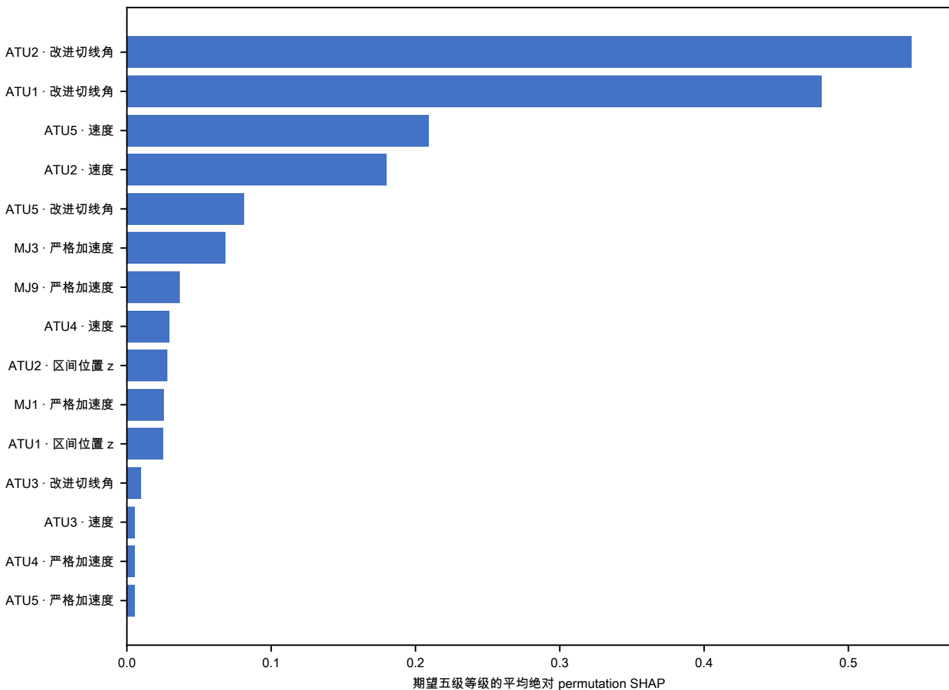
第 2 时间折：滑坡体级 NGBoost 的模型依赖（非因果）
