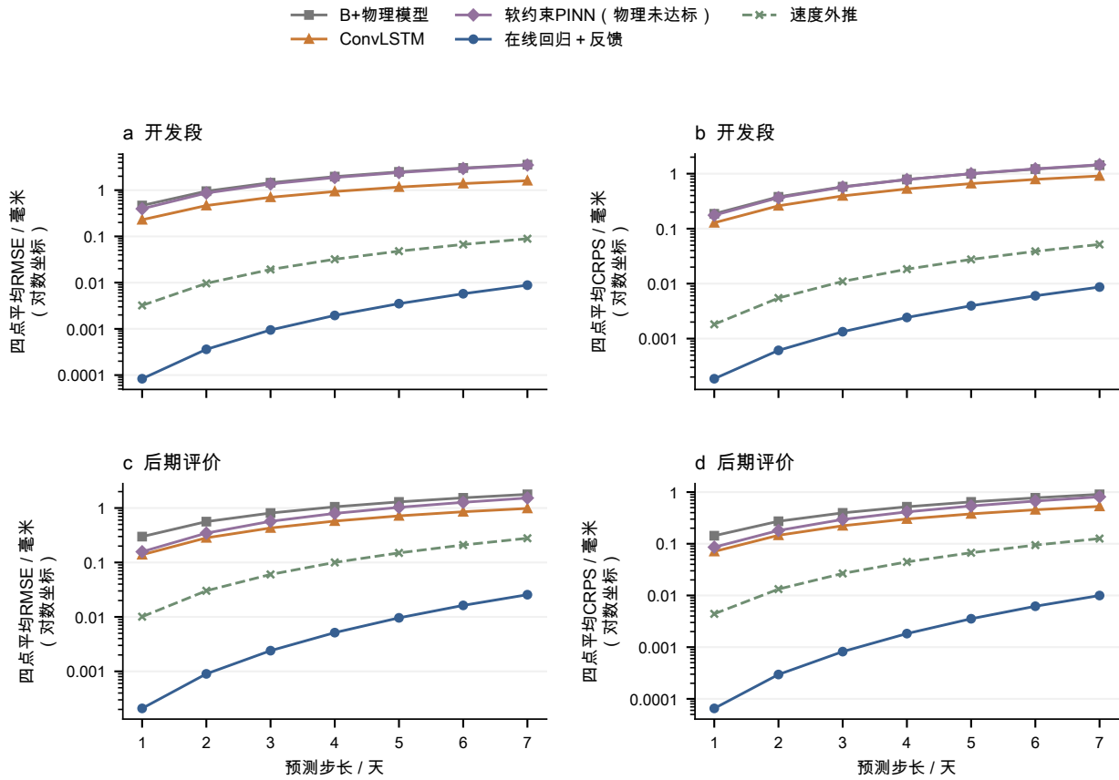
图 1 同一步长比较同一组起点。各类代表按开发 RMSE 选择，后期沿用；纵轴为对数。
