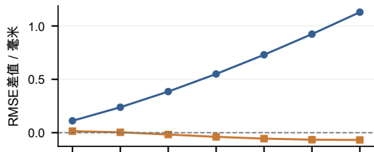
a ConvLSTM : 残差 - 直接
