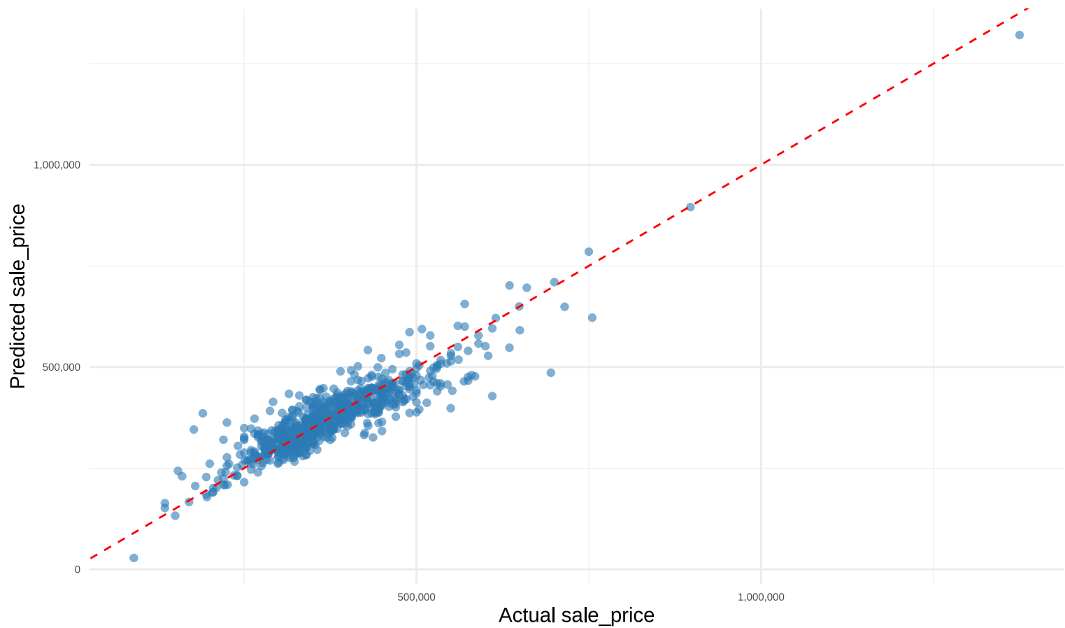
Actual vs Predicted
