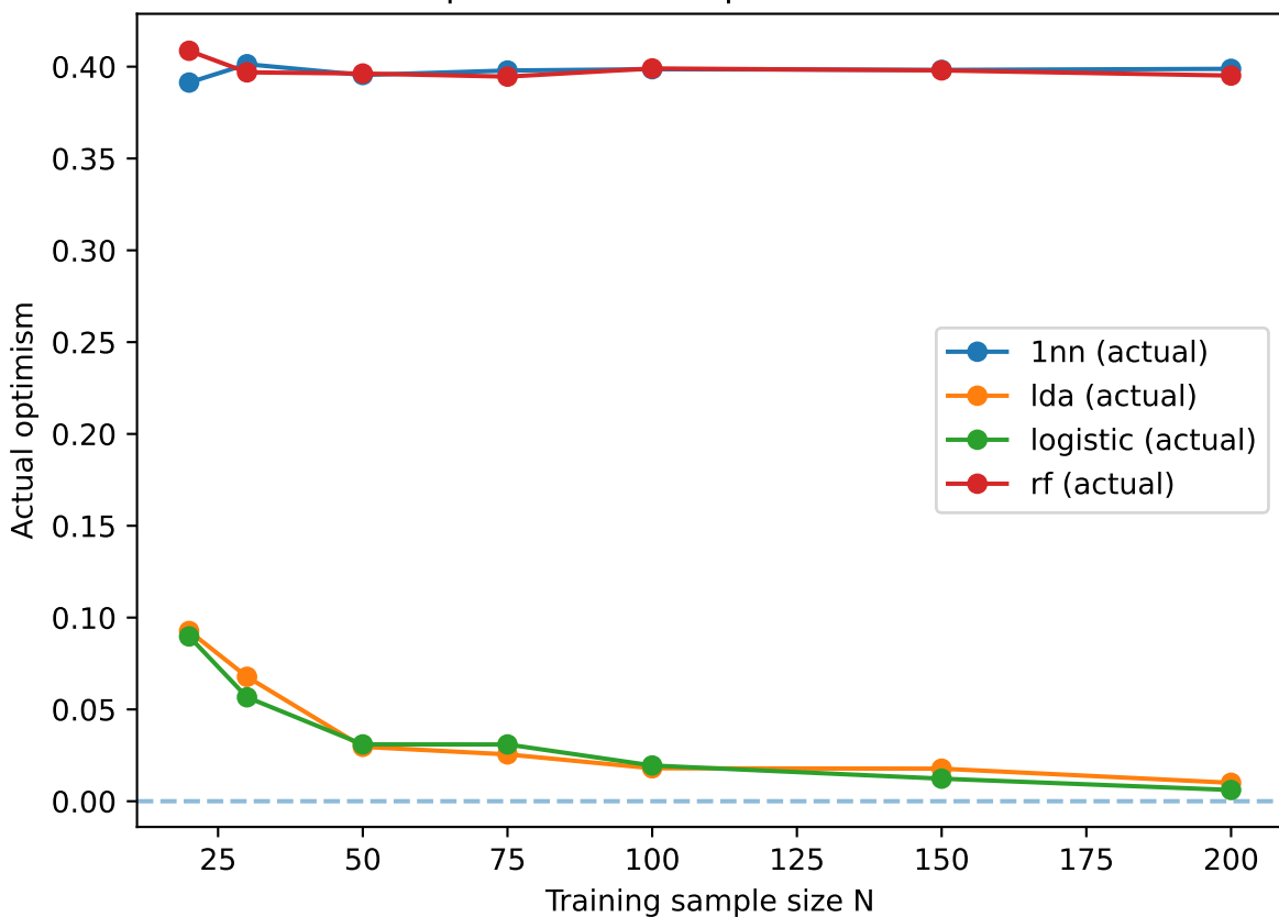
Actual optimism vs sample size for DGP: efron
