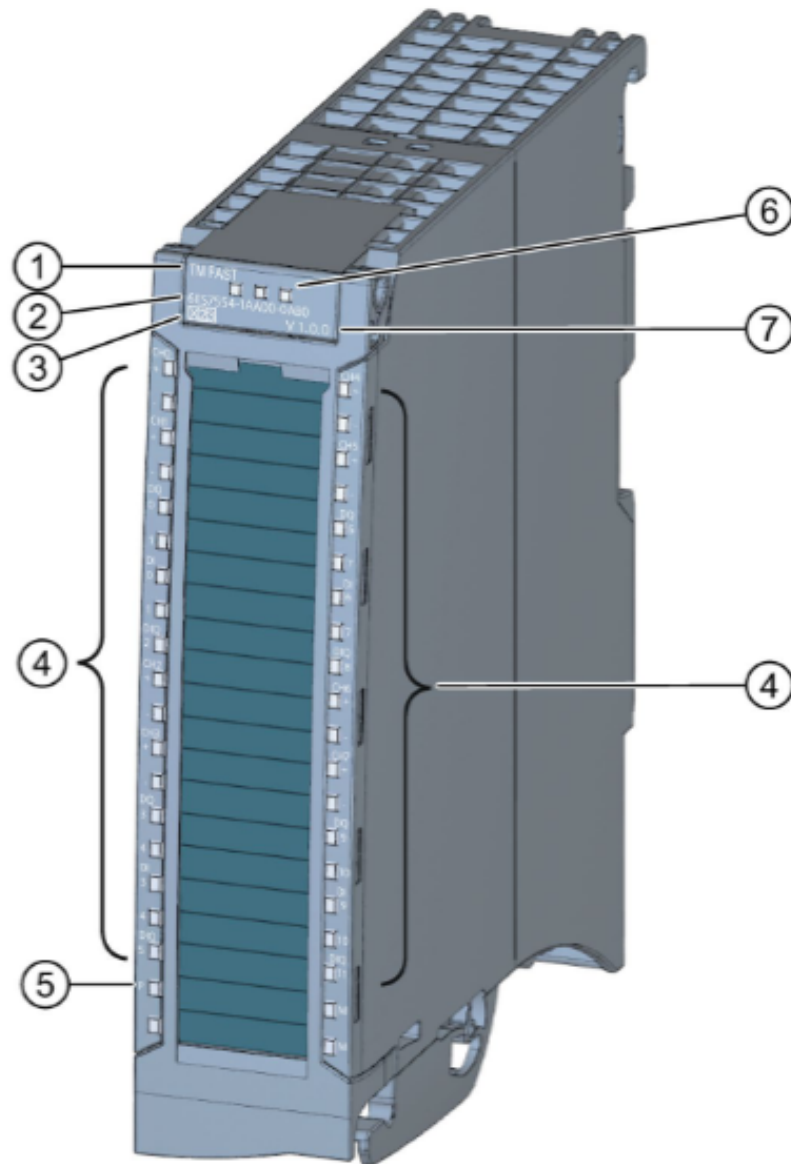
Abbildung 3.5: Abbildung 8: Technologiemodul TM FAST [8]
