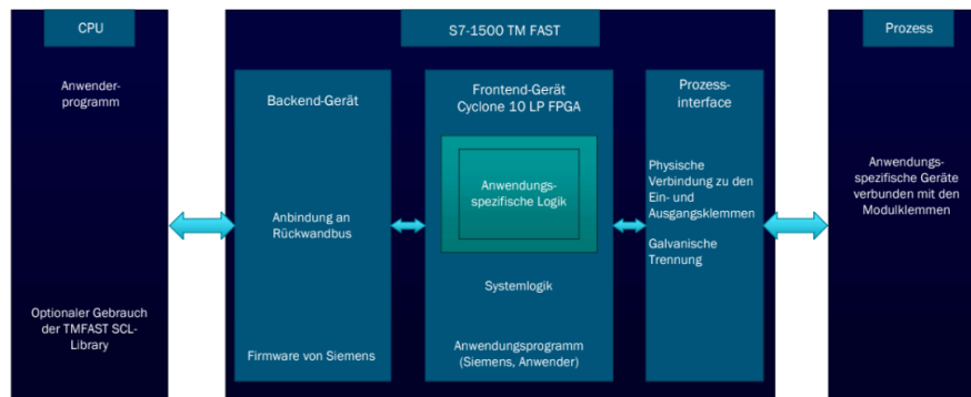
Abbildung 3.2: Abbildung 6: Aufbau des TM FAST als Blockdiagramm [Guillaume: Specification for TM Fast]
