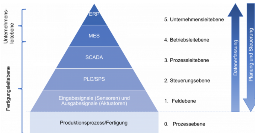
Abbildung 2.1: Abbildung 1: Automatisierungspyramide, Quelle: IPH Hannover, https://www.iph-hannover.de/de/dienstleistungen/automatisierungstechnik/automatisierungspyramide/ , abgerufen am 26.07.2025
