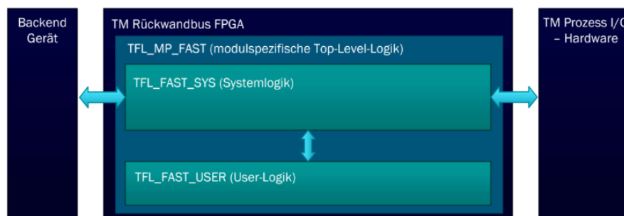
Abbildung 3.3: Abbildung 7: Aufbau aus Backend- und Frontend-Gerät und Zusammensetzung der Logik des TM FAST [Guillaume: Specification for TM Fast]
