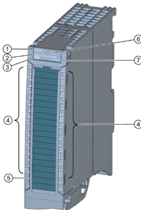
Abbildung 3.3: Technologiemodul TM FAST [3]
