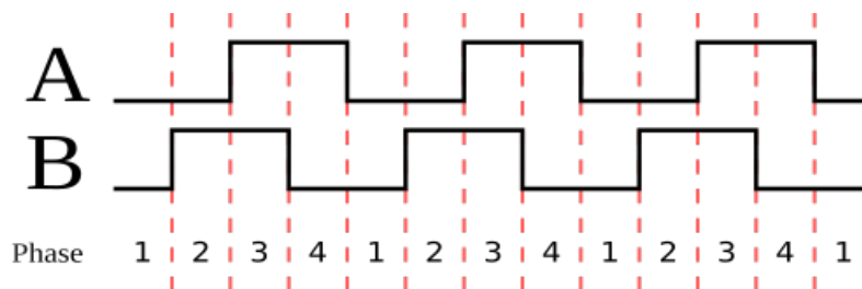
Abbildung 2.6: Zwei Rechteckwellen in Quadratur [12]
