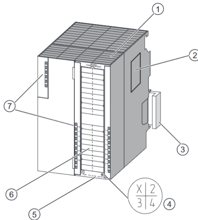
Abbildung 3.5: Hardware der FM-350-2 [7]
