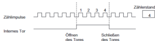
Abbildung 3.11: Öffnen und Schließen eines Tores und das Zählen der Impulse [7]
