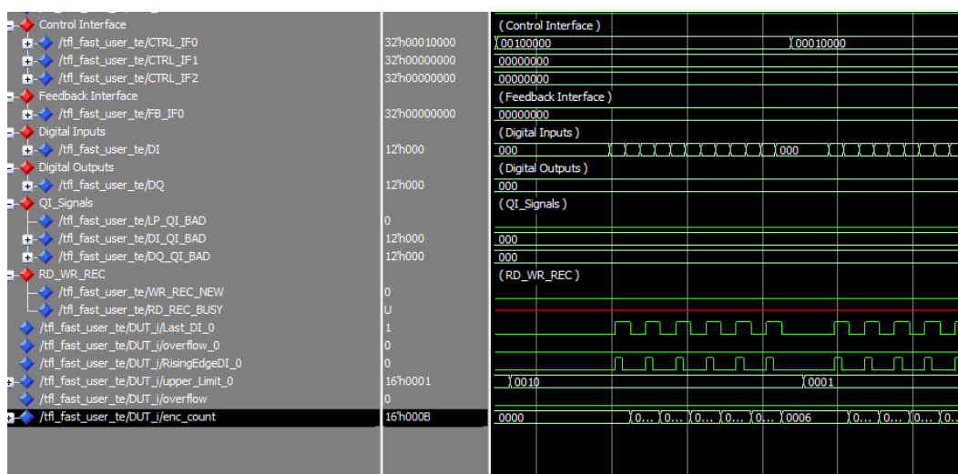
Abbildung 4.3: Wellenanalyse der CTRL_IF-, WR_REC- und RD_REC-Schnittstellen in Questa
