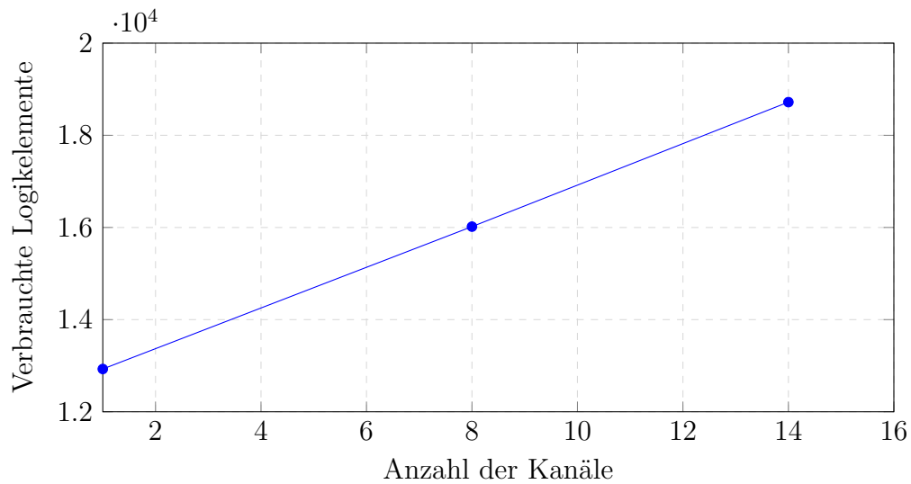
Abbildung 4.5: Verbrauchte Logikelemente in Abhängigkeit von der Kanalanzahl
