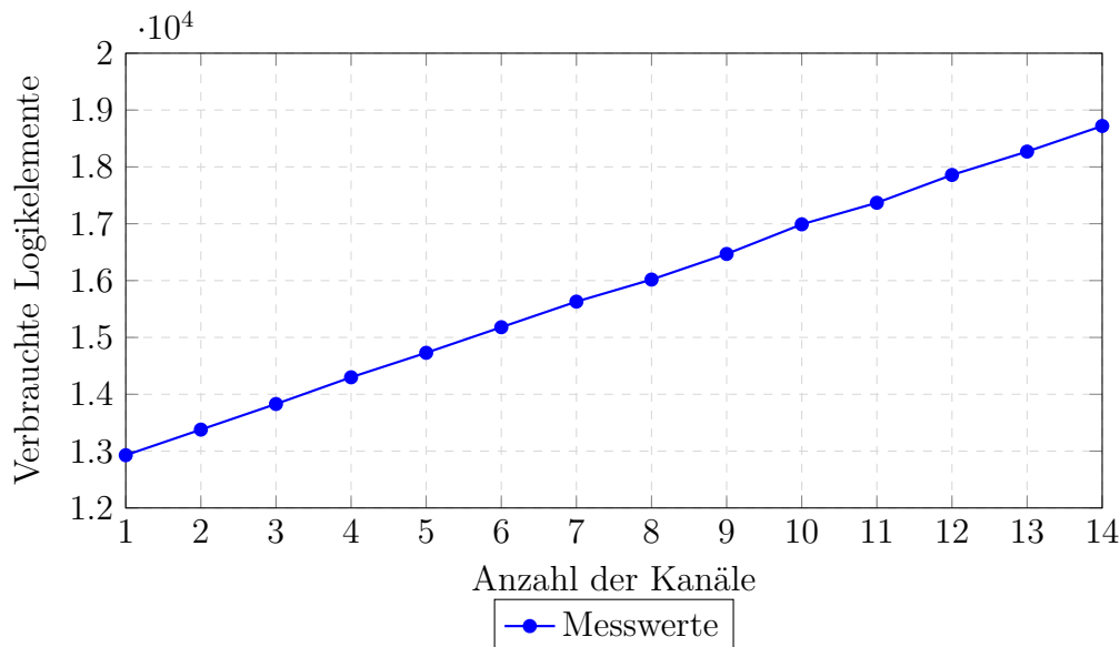
Abbildung 4.2: Verbrauchte Logikelemente in Abhängigkeit von der Kanalanzahl
