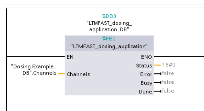
Abbildung 4.4: Integration des Applikationsbausteins in OB1
