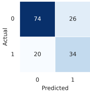
Gaussian NB
