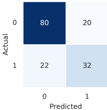
MLP
