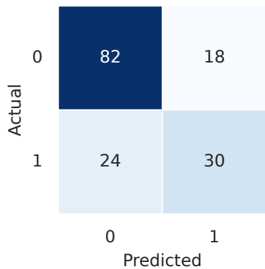
Gaussian NB
