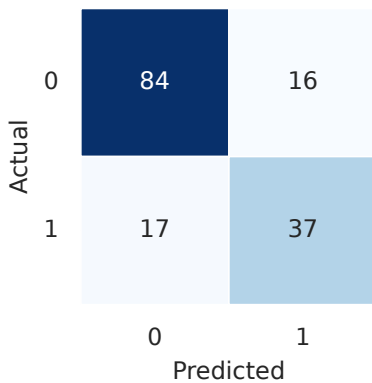
MLP
