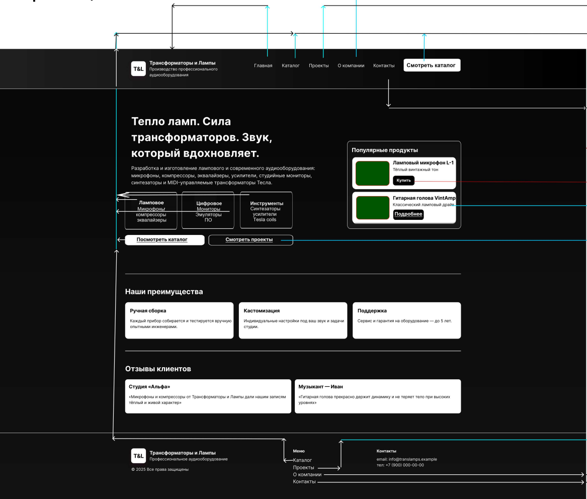
Страница index.html
