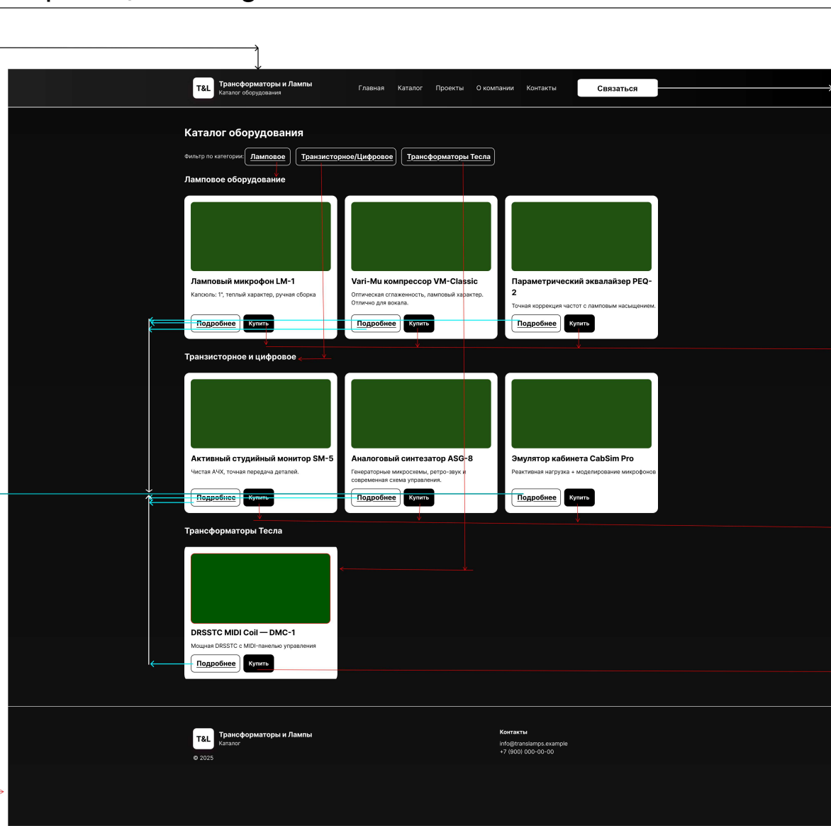
Страница catalog.html
