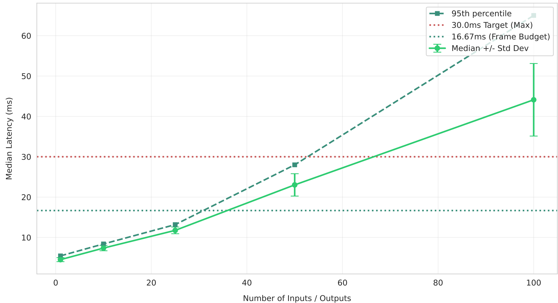
E2E Latency vs Input Count
