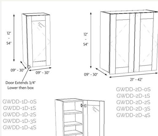
Wall Cabinet, 1 Door
