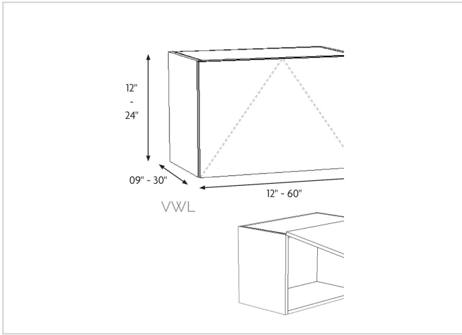
Wall Cabinet, 1 Door
