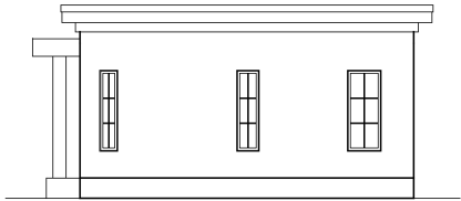
Right Elevation
