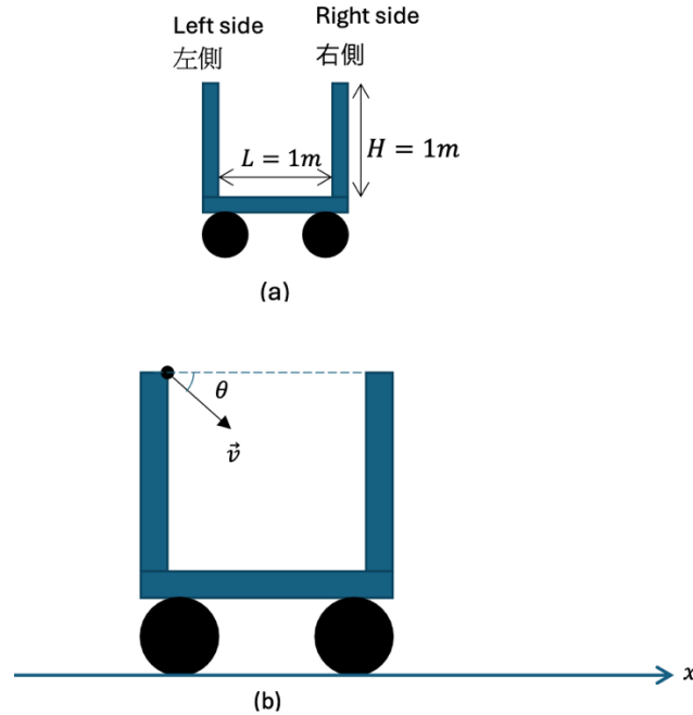
Figure 3: (a) Dimension of the trolley basket. (a) 手推車籃的尺寸。 (b) A particle enters the basket at the top left corner with a velocity \vec{v} . (b) 一個粒子以速度矢量 \vec{v} 從左上角進入籃子。
