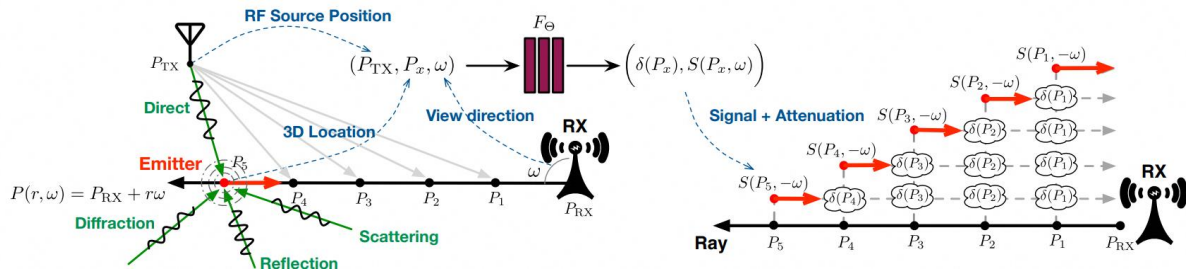
图4 基于NeRF的无线数字孪生[4]
