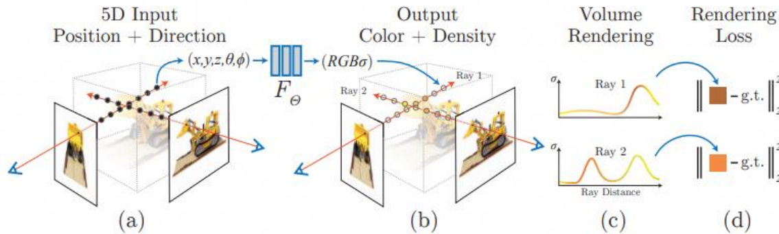
图2 NeRF技术[2]
