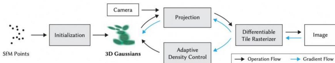
图3 3DGS技术[3]
