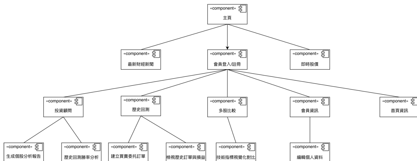
▲圖 7-3-1 元件圖
