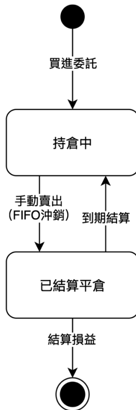
▲圖 7-4-2 模擬下單之狀態機圖
