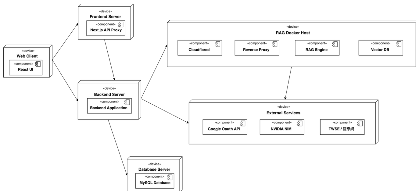
▲圖 7-1-1 佈署圖
