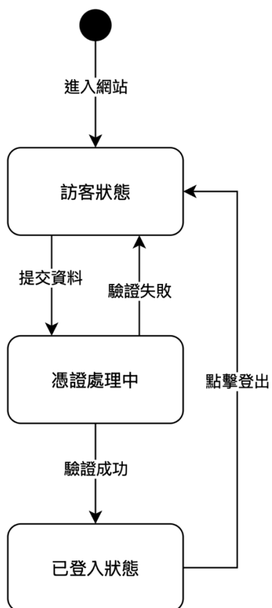
▲圖 7-4-1 會員登入/註冊之狀態機圖
