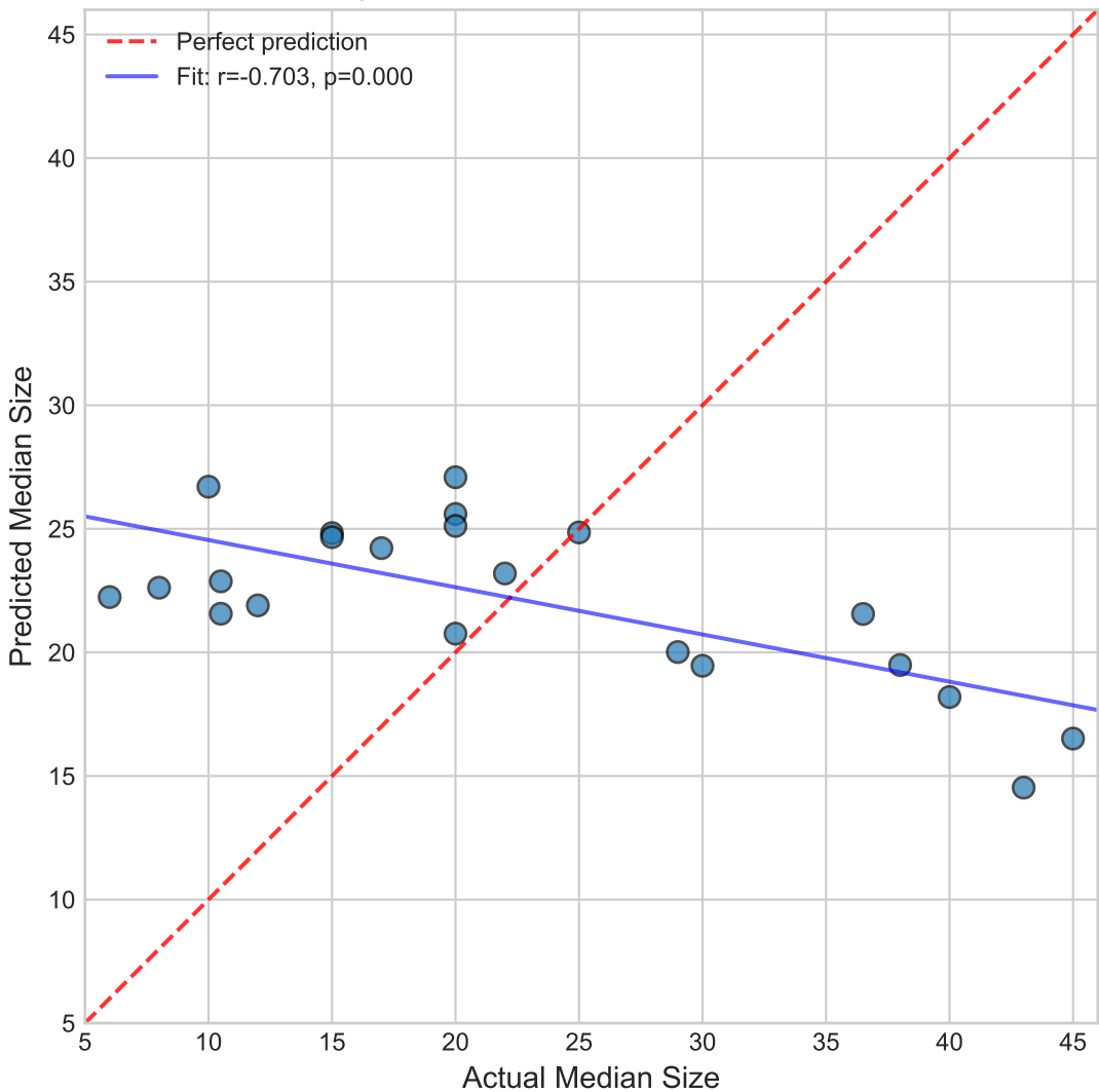
Ridge: Predicted vs Actual Median Size
