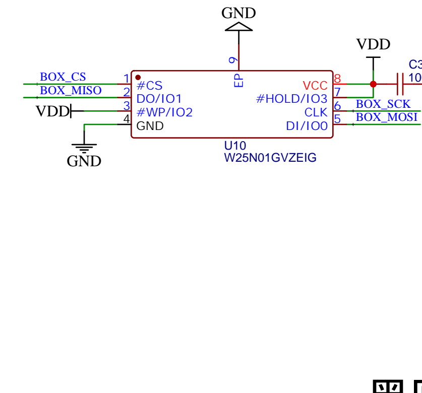
黑匣子
