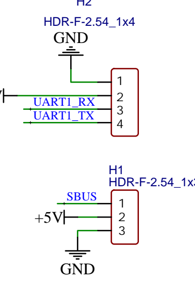
Reciver 接收机
