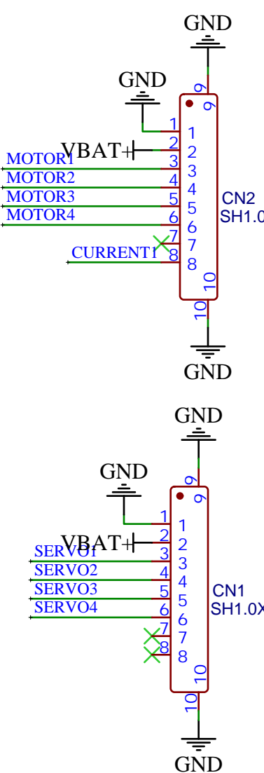
接飞控
