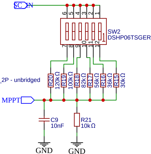
MPPT Setpoint Circuit 4.5V Vmpp 5.5V Vmpp 12.2v Vmpp 16.9v Vmpp
