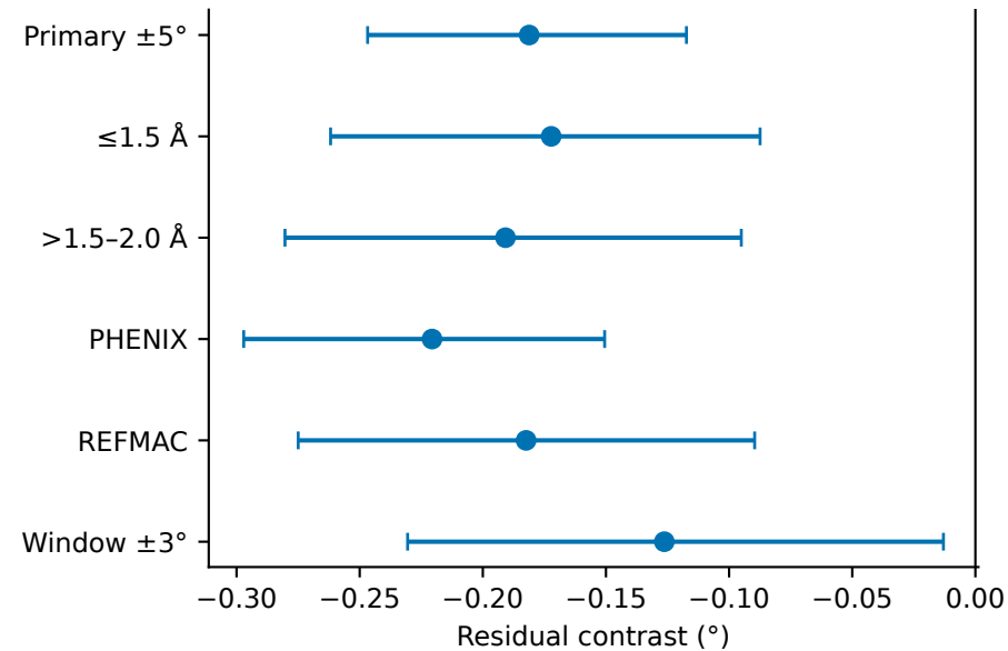
E PPII robustness
