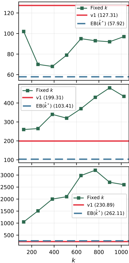
TPOT p99 (ms)
